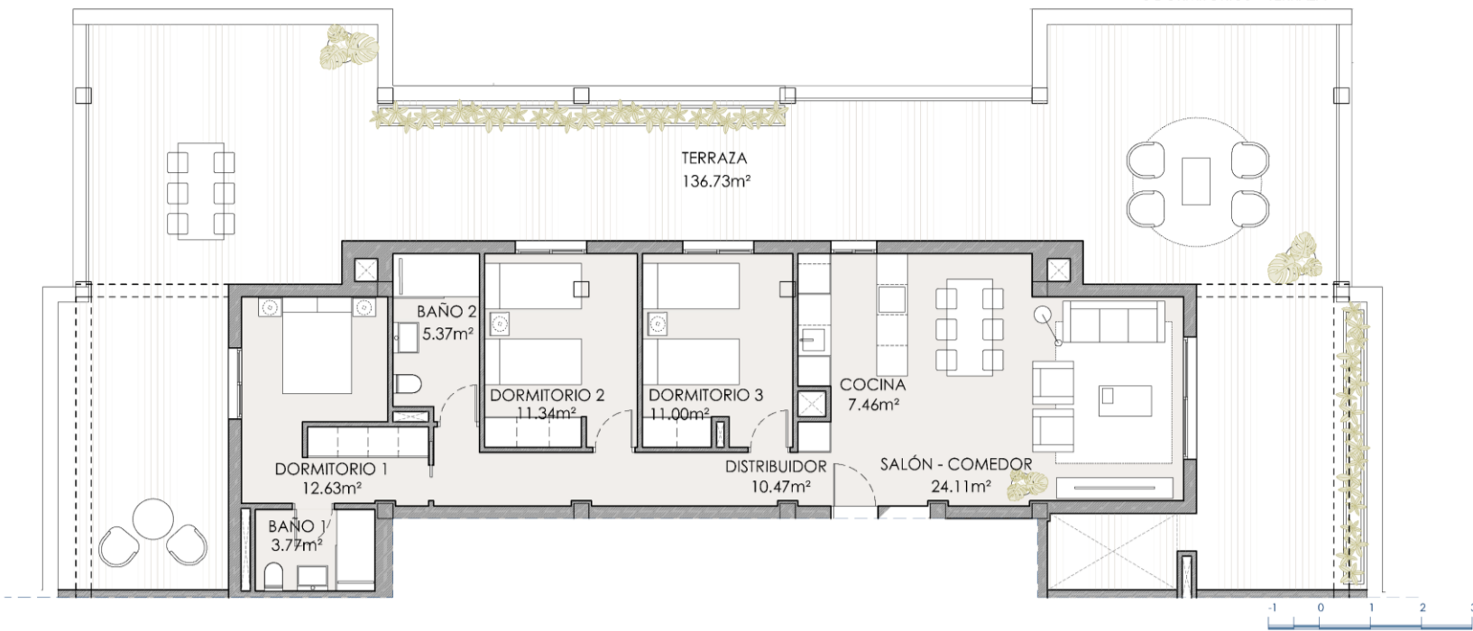
VIVIENDA ÁTICO °A 3 DORMITORIOS + TERRAZA
