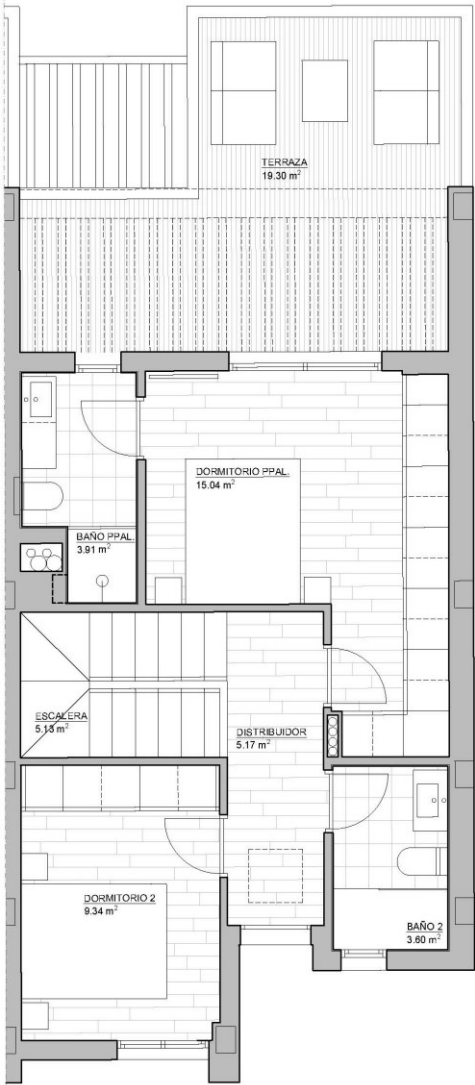
PLANTA PRIMERA
