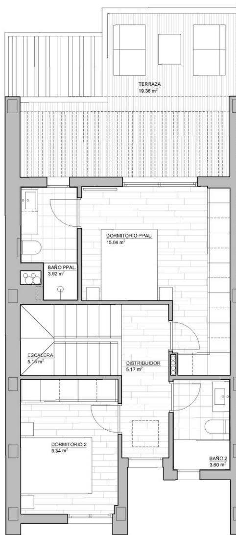
PLANTA PRIMERA
