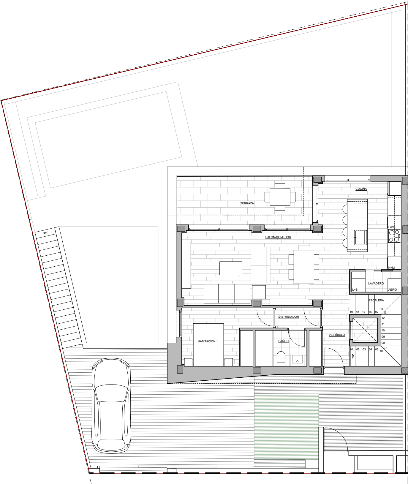
PLANTA PRIMERA
