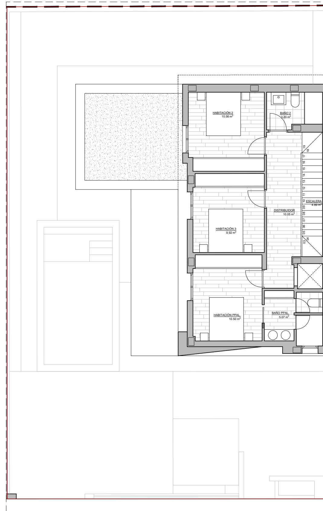
PLANTA PRIMERA
