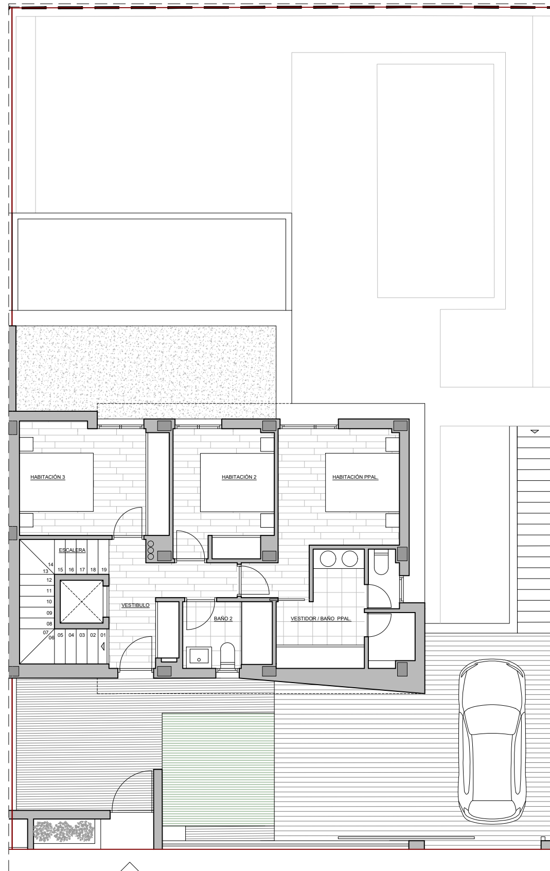
PLANTA PRIMERA
