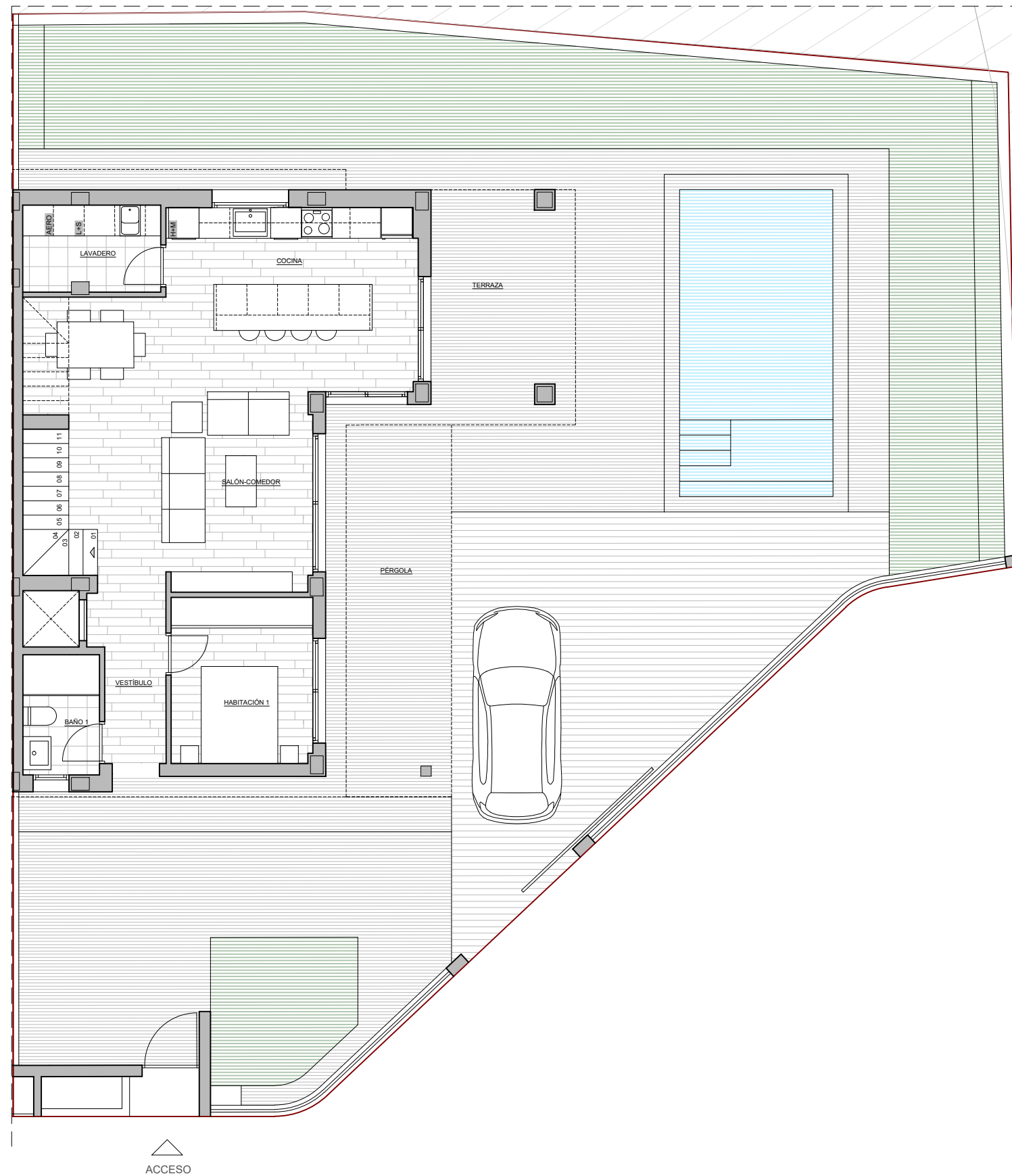
PLANTA BAJA
