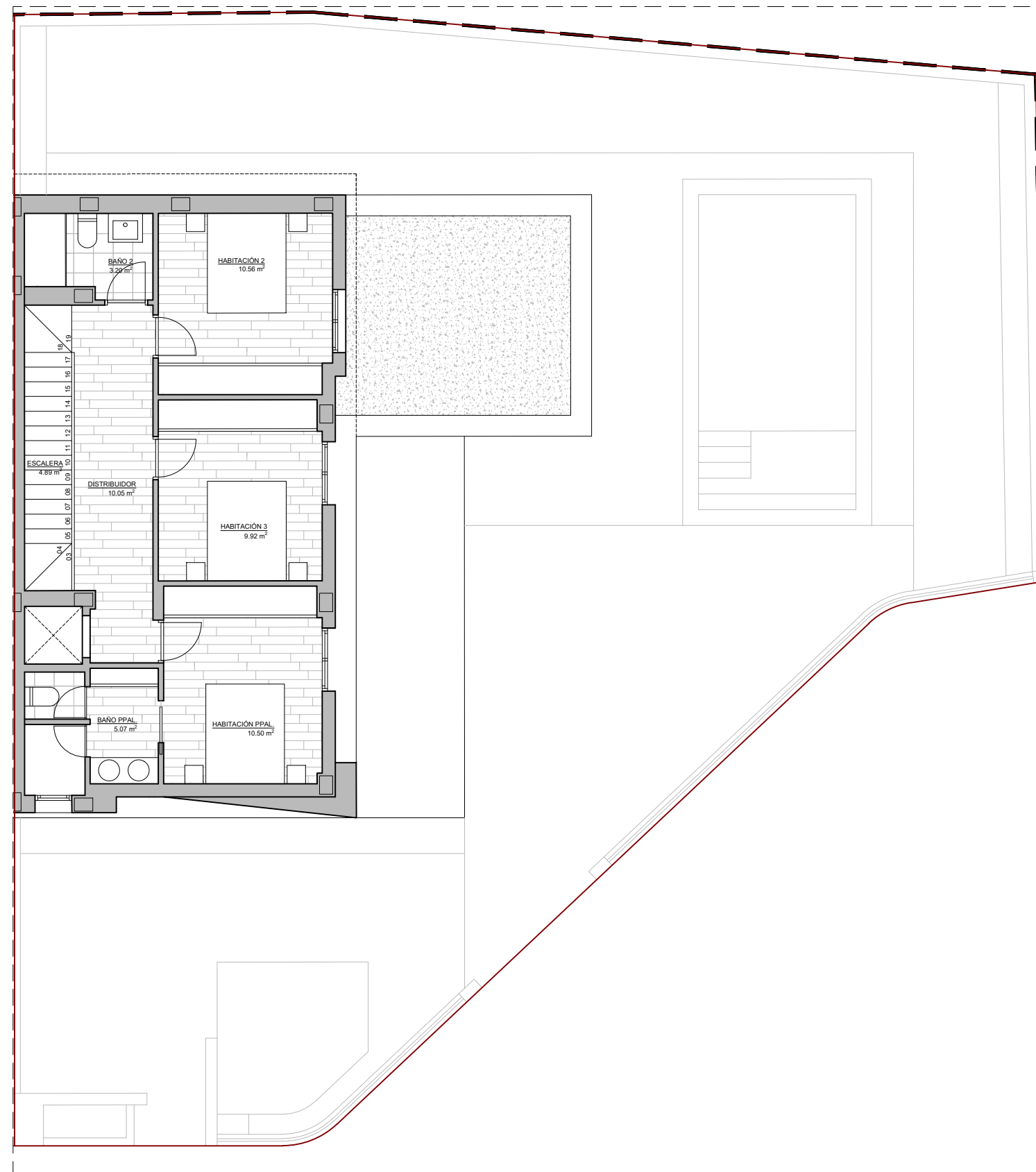
PLANTA PRIMERA
