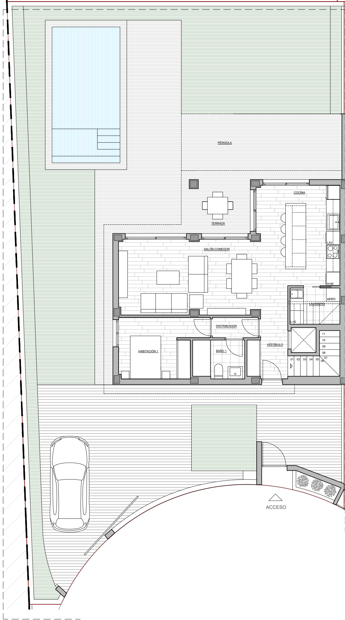
PLANTA BAJA
