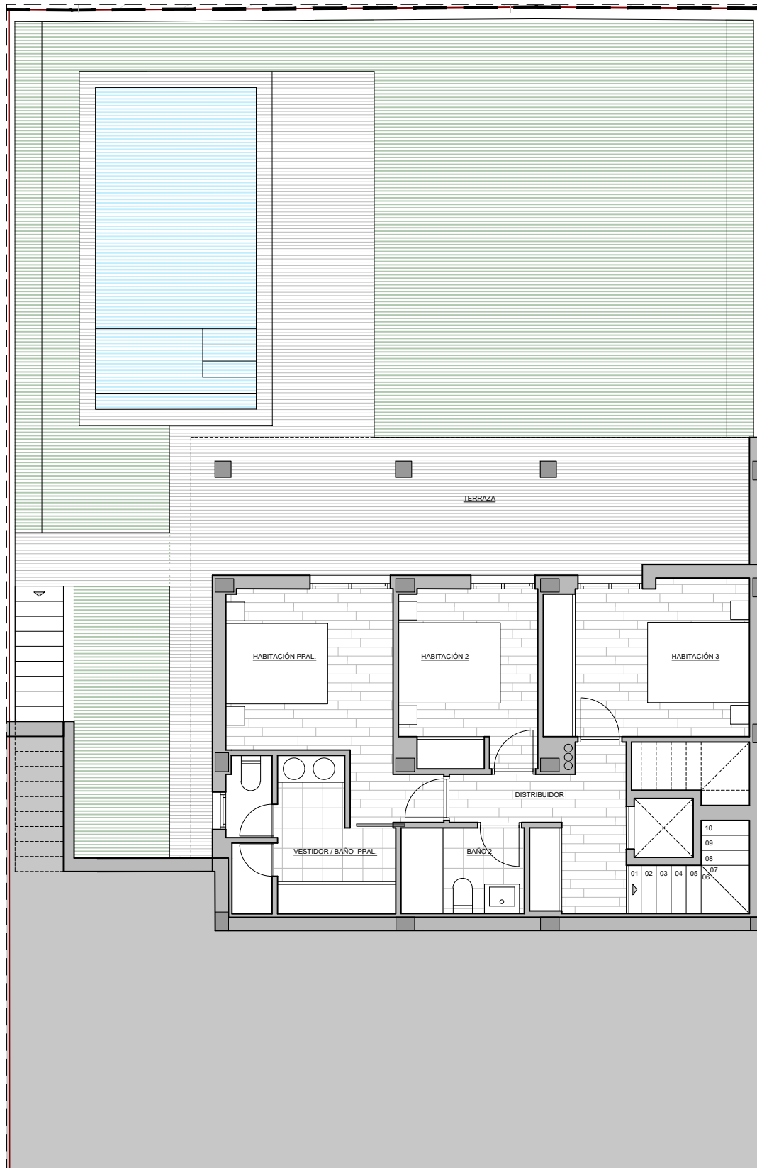
PLANTA BAJA
