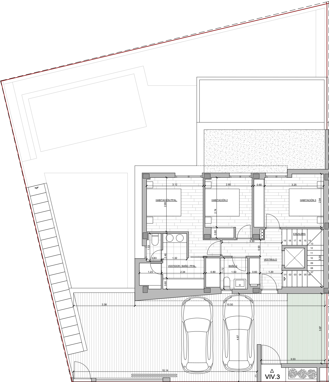
PLANTA PRIMERA
