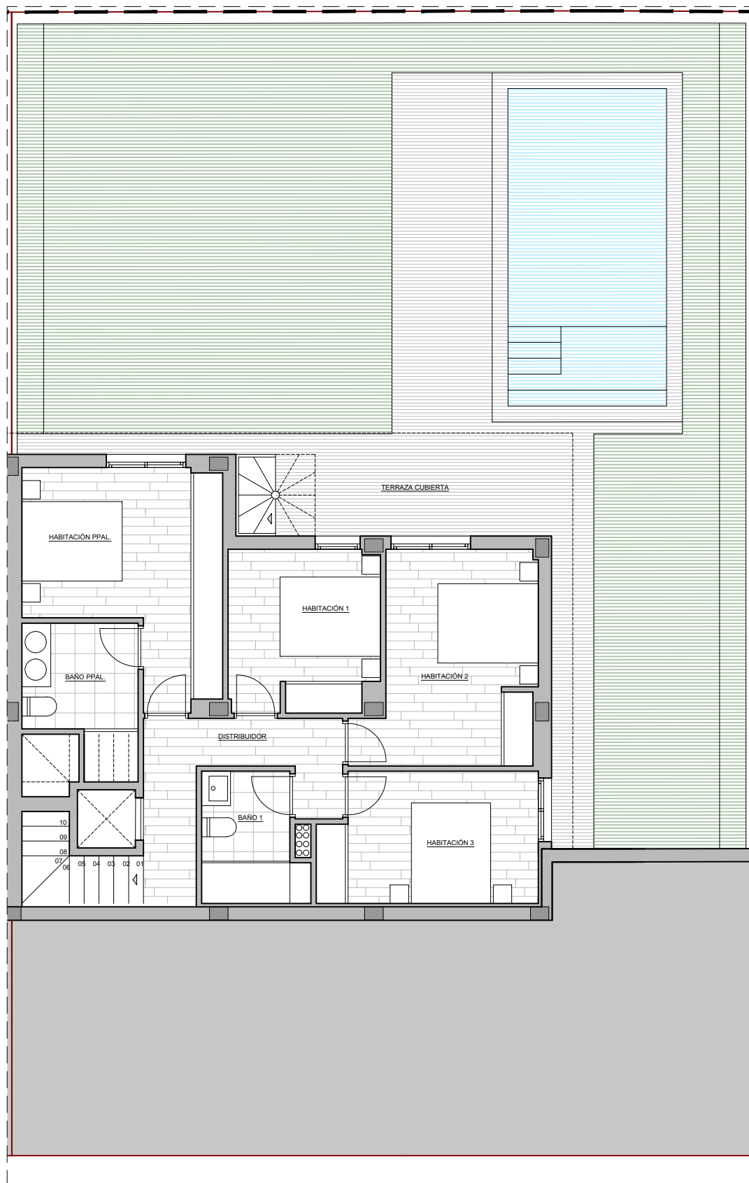
PLANTA BAJA
