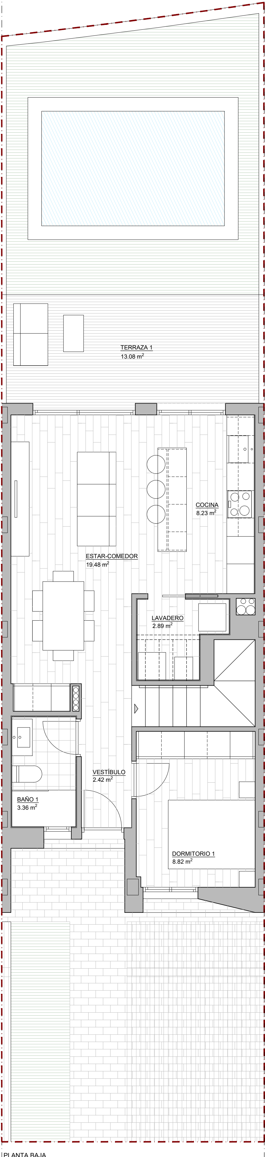
PLANTA BAJA
