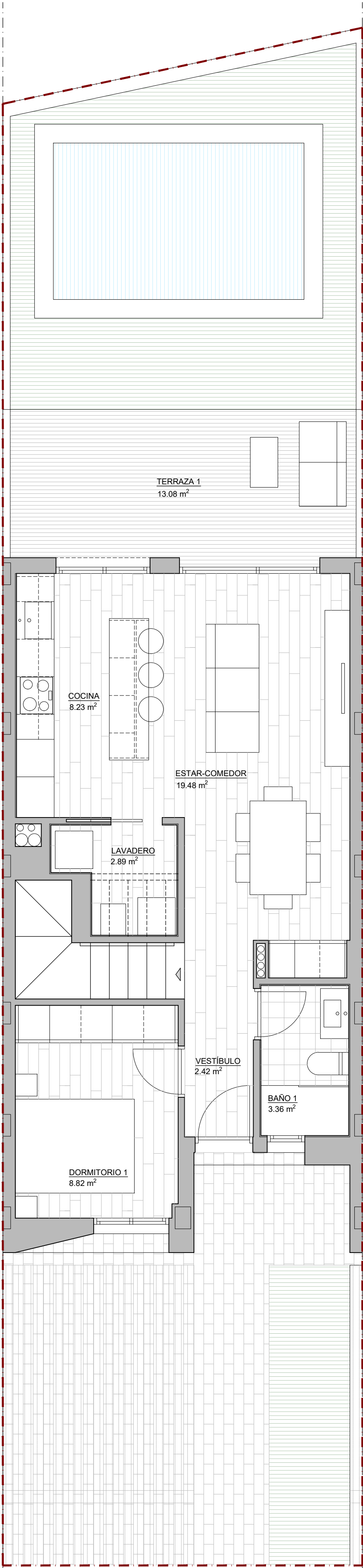
PLANTA BAJA
