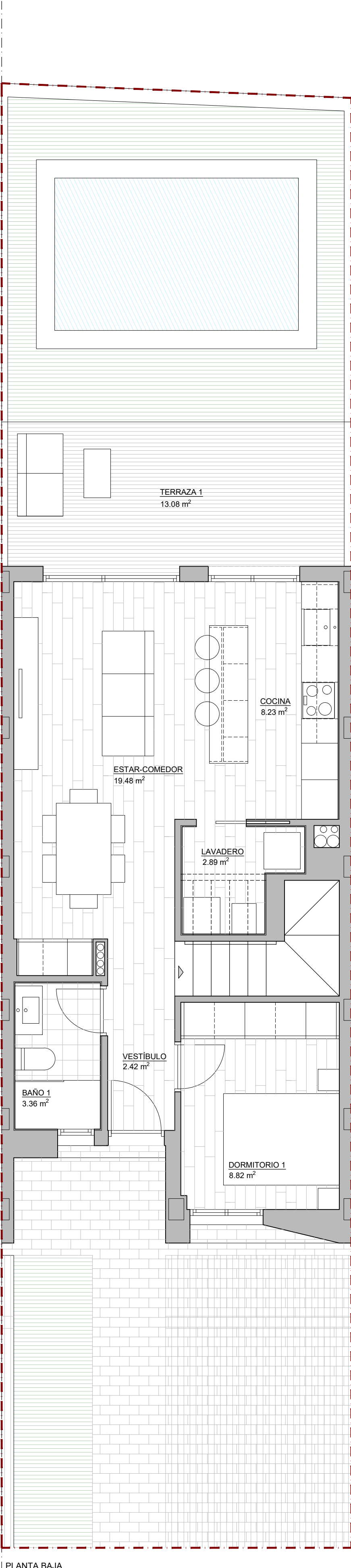
PLANTA BAJA
