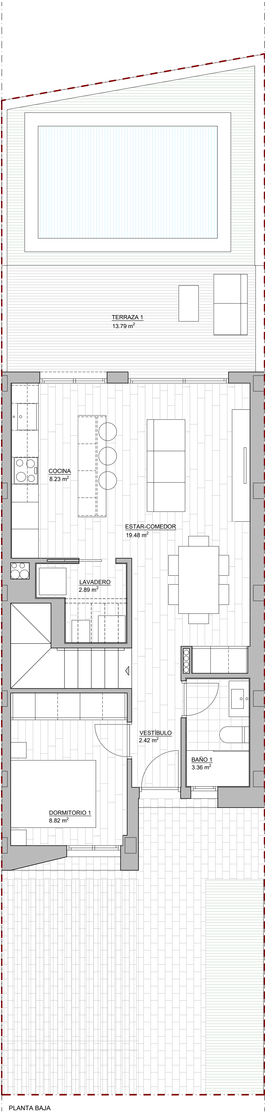
PLANTA BAJA
