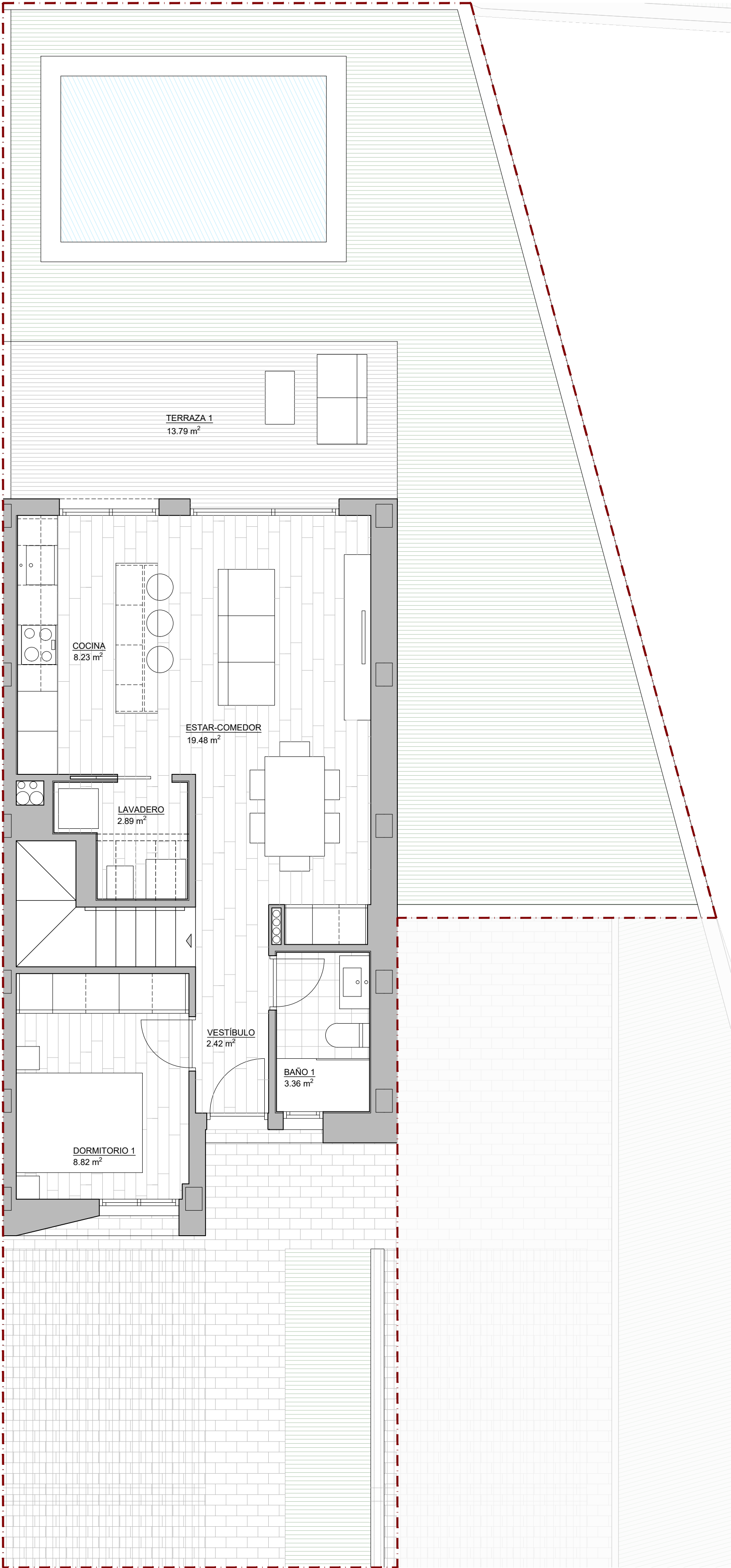
PLANTA BAJA
