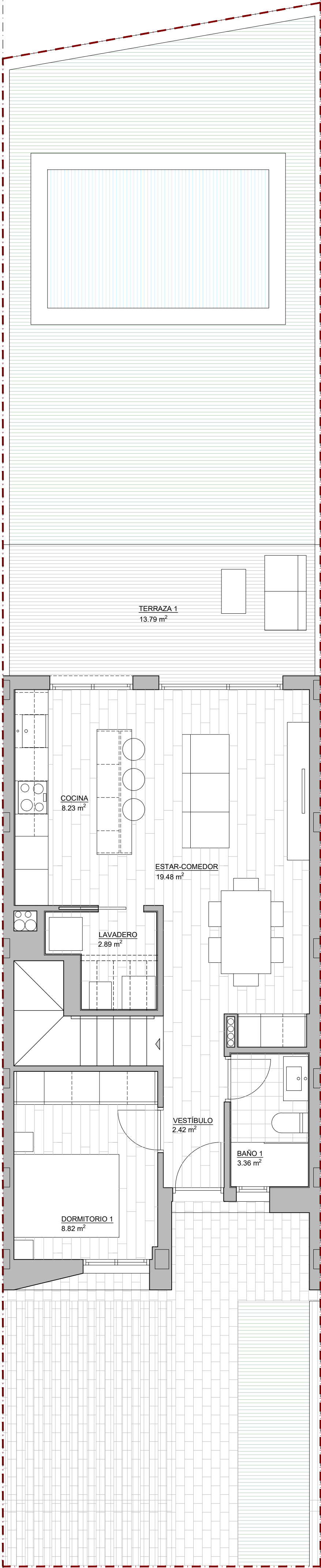
PLANTA BAJA
