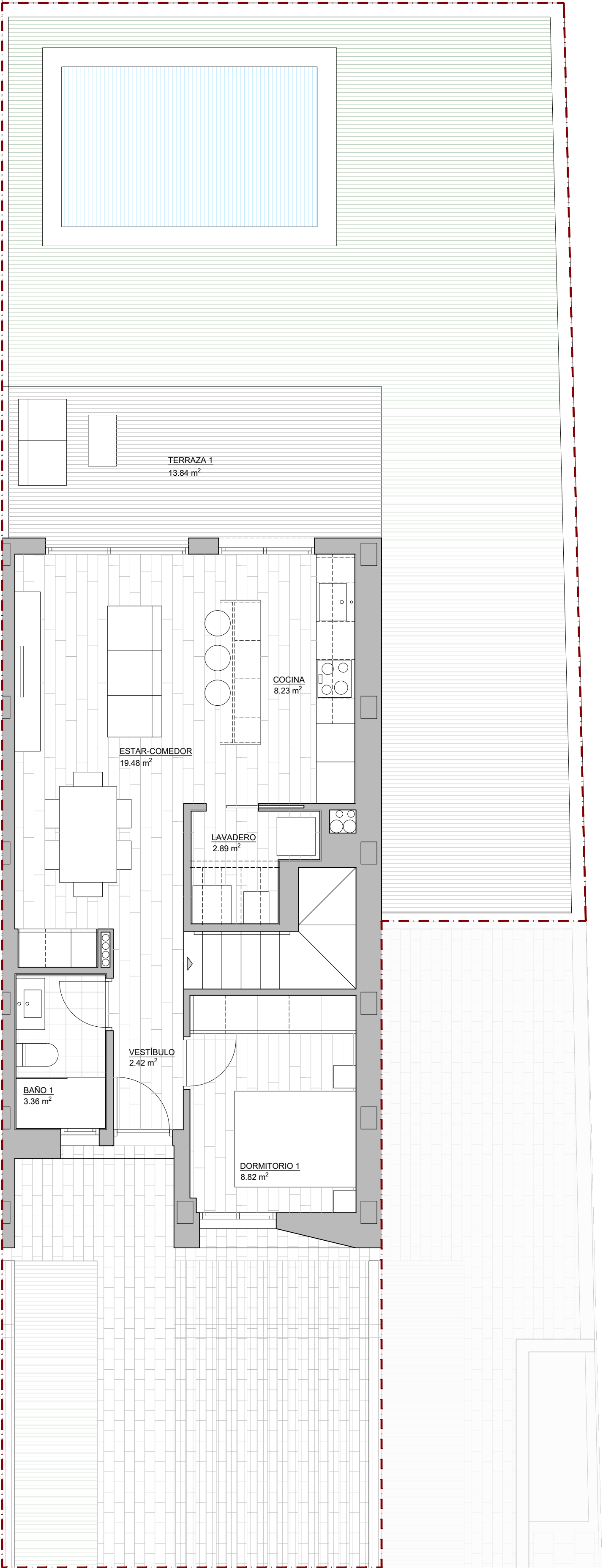
PLANTA BAJA
