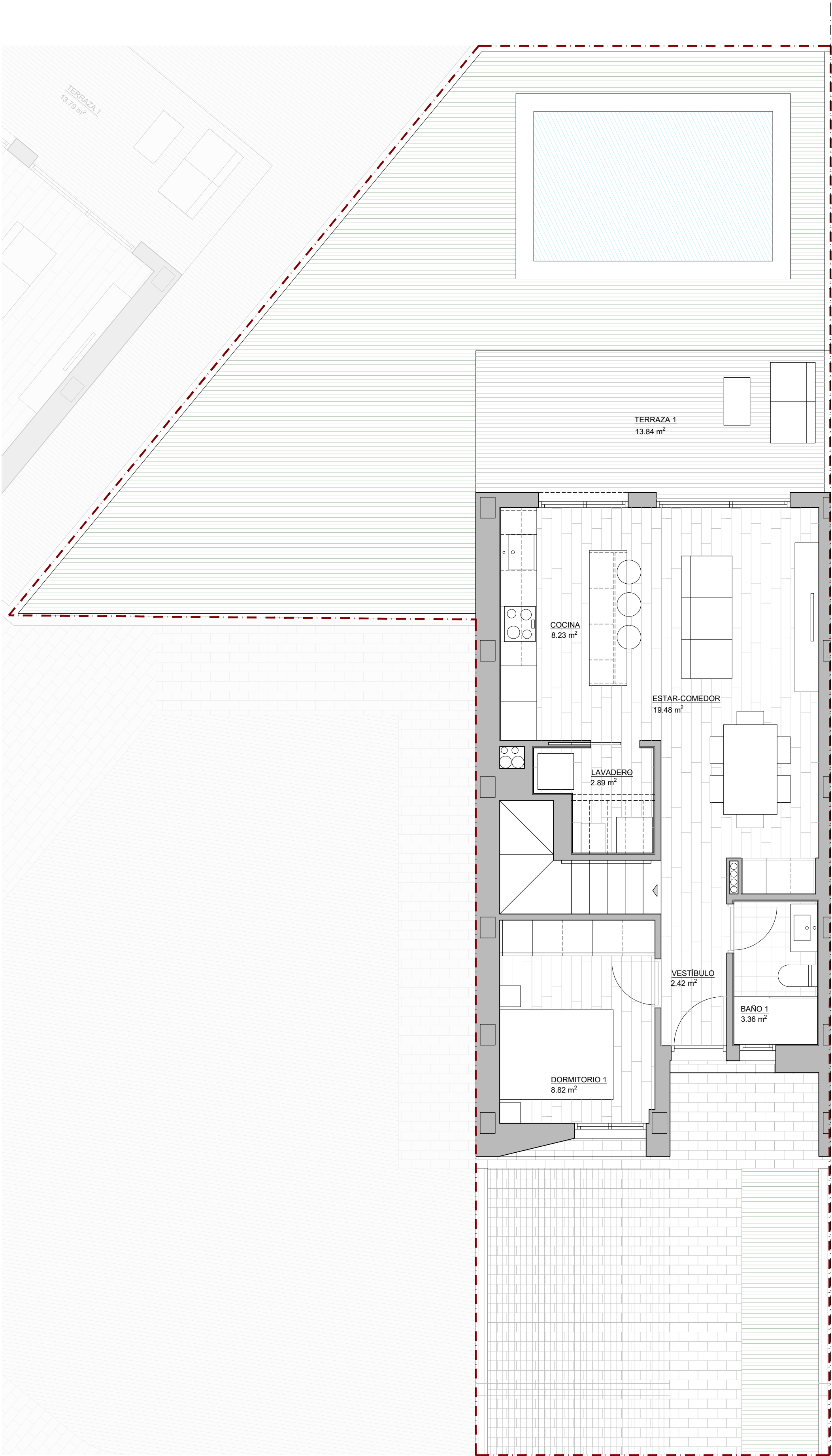
PLANTA BAJA
