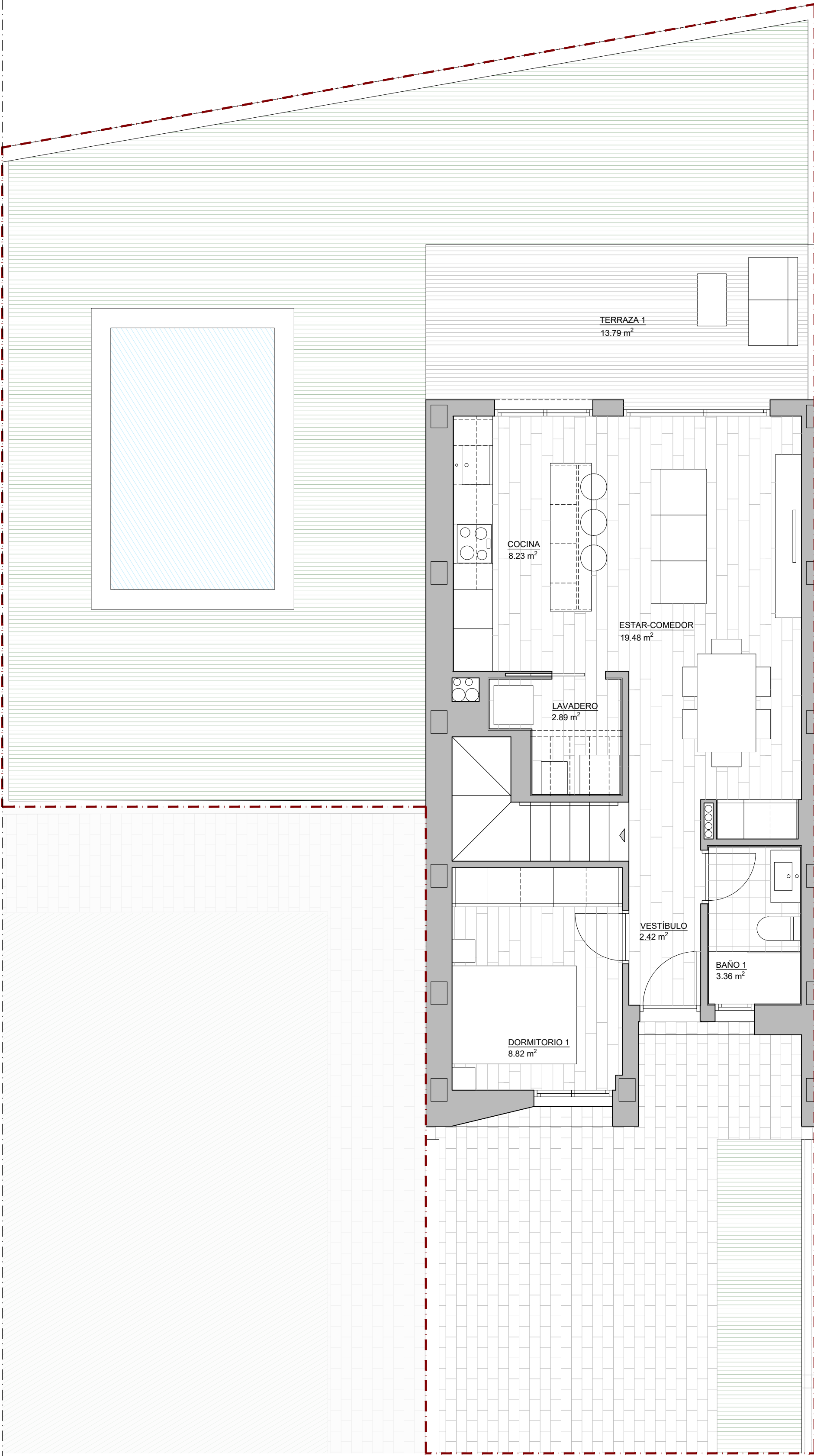
PLANTA BAJA
