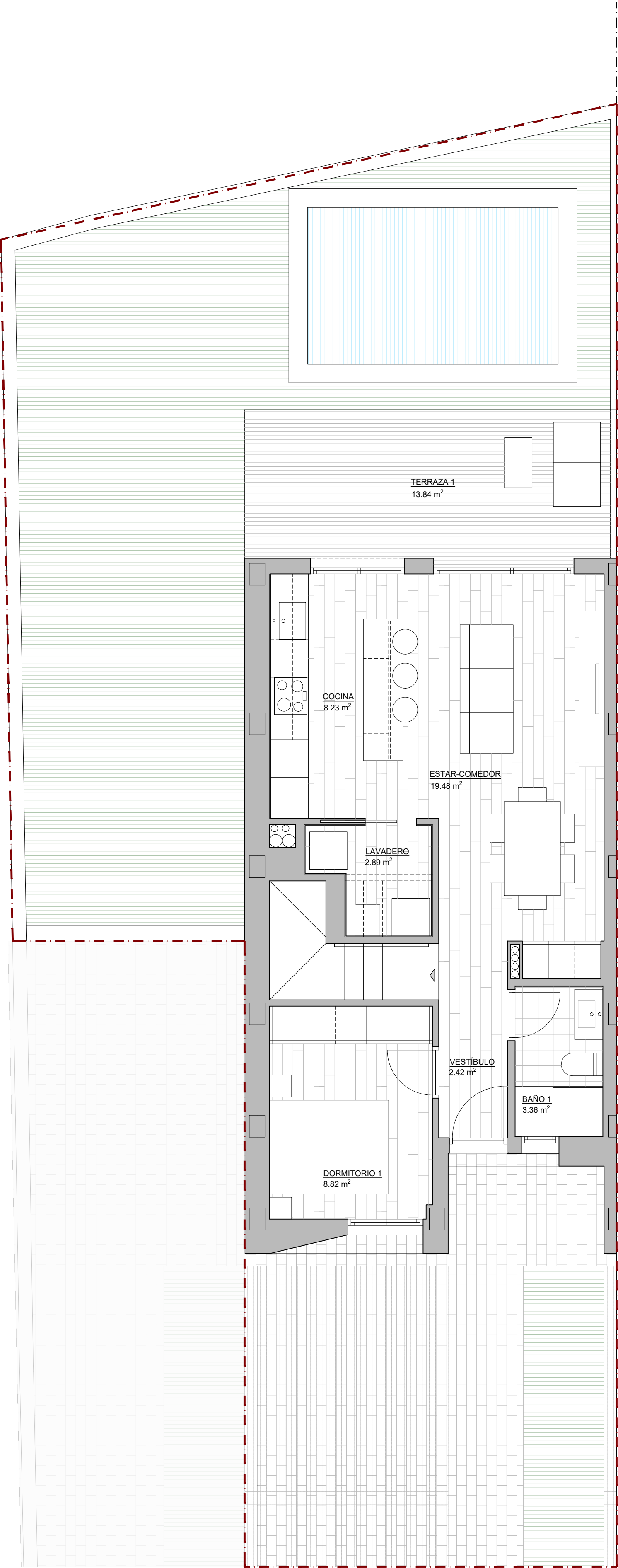
PLANTA BAJA
