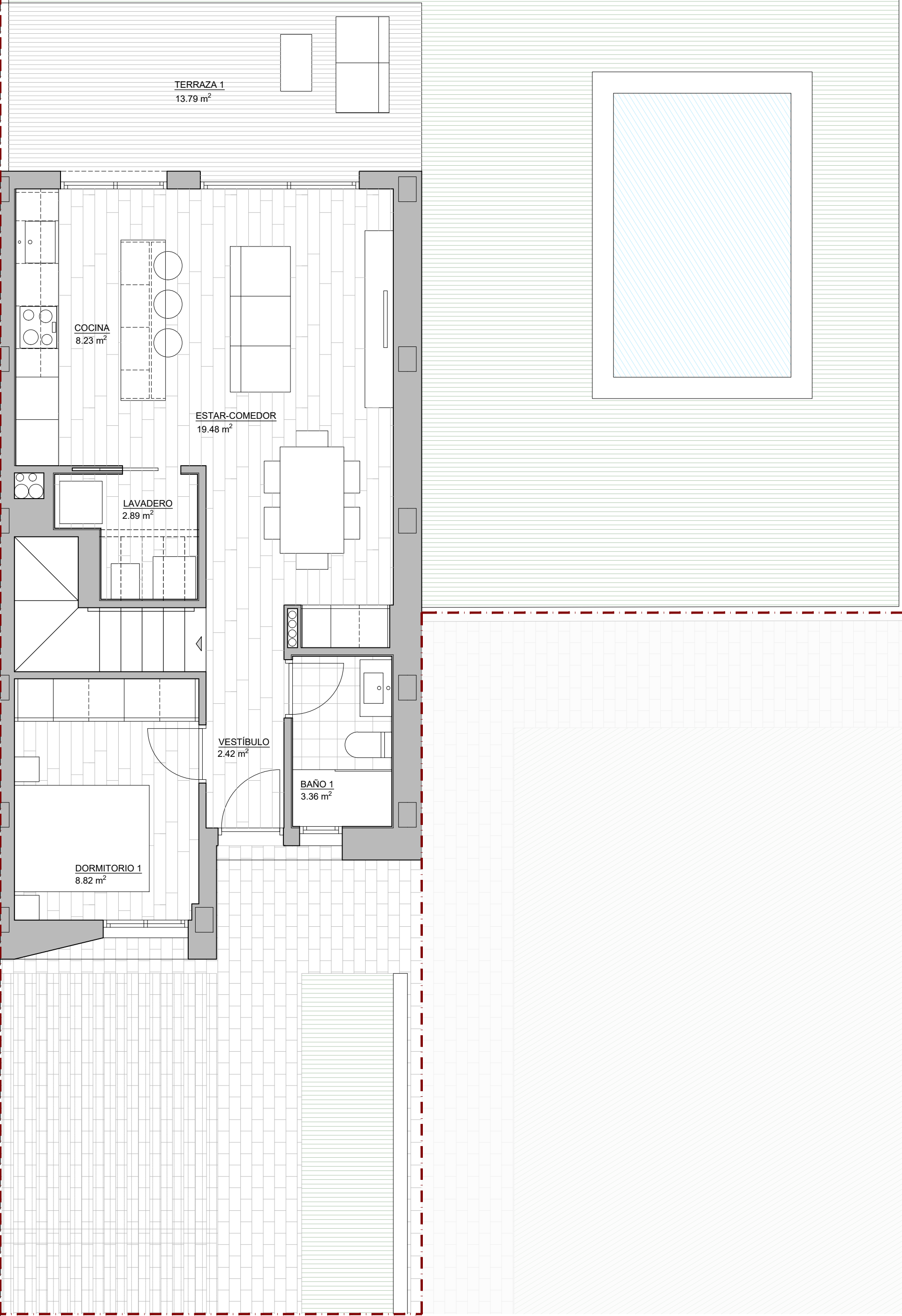
PLANTA BAJA
