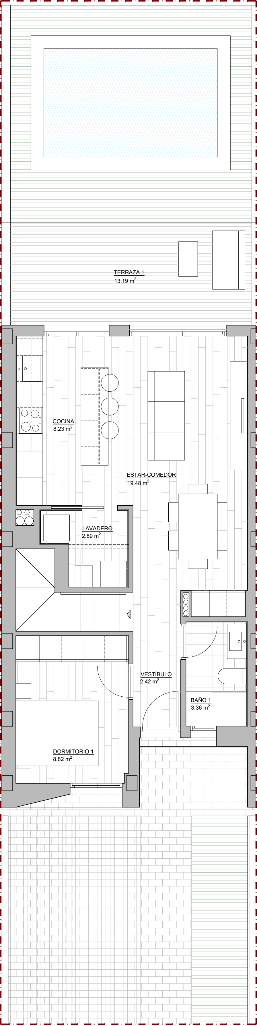
PLANTA BAJA
