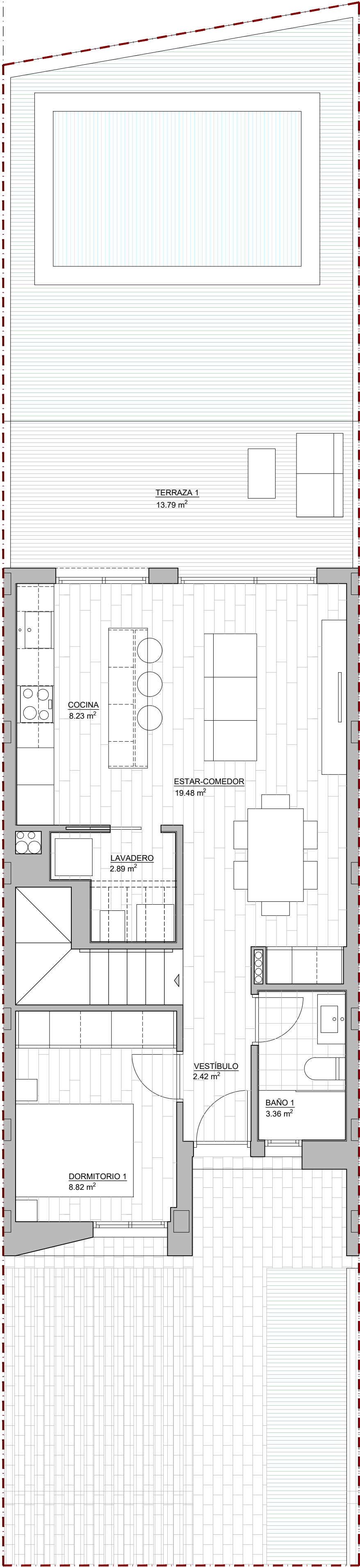
PLANTA BAJA
