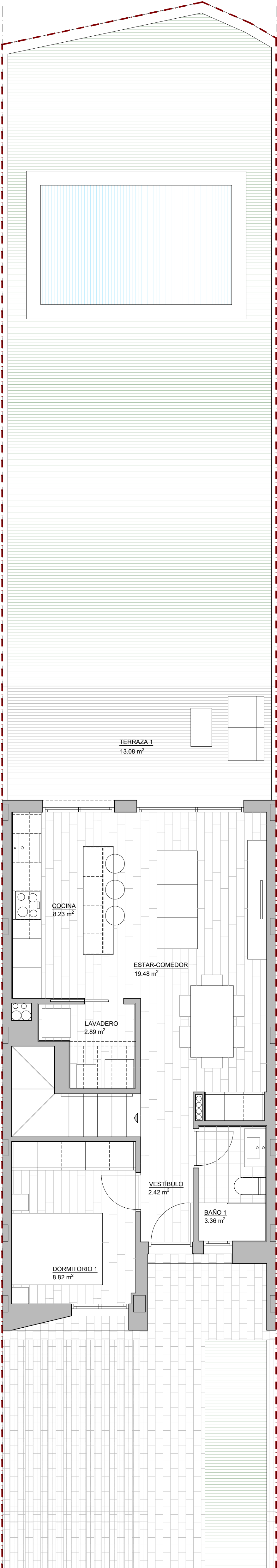
PLANTA BAJA
