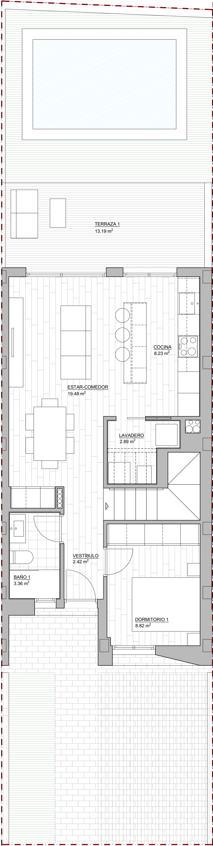
PLANTA BAJA
