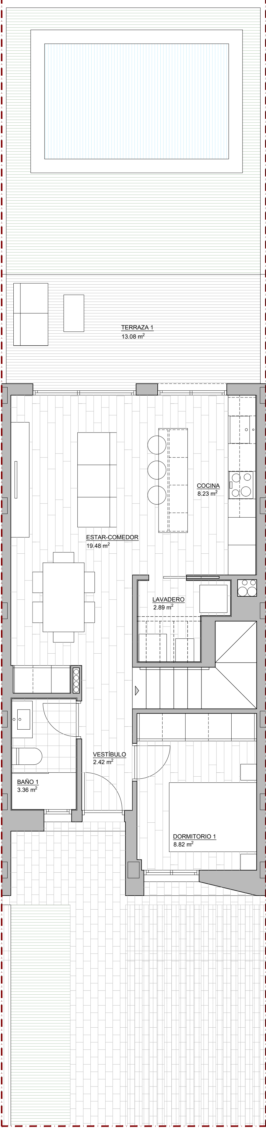
PLANTA BAJA
