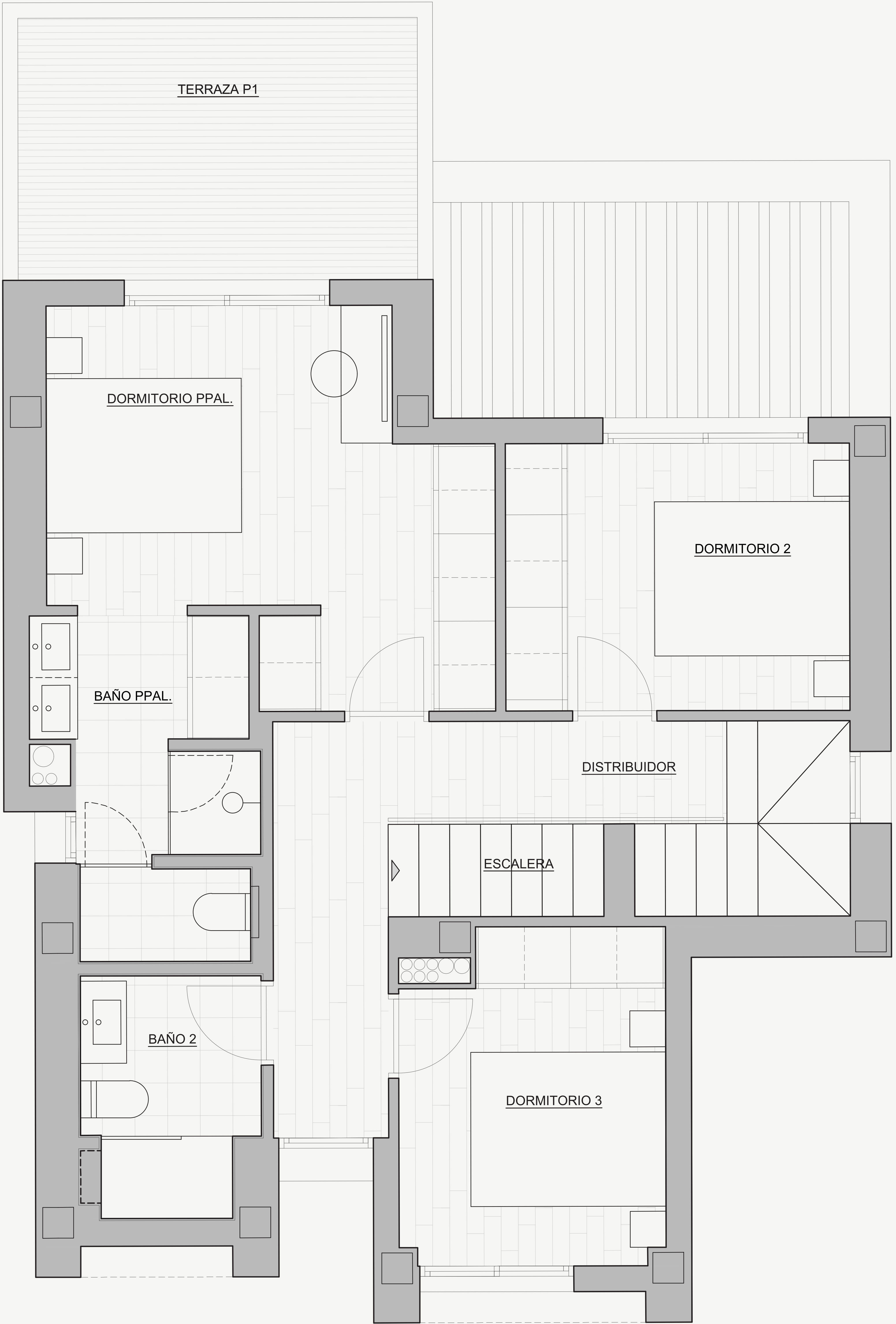
PLANTA PRIMERA
