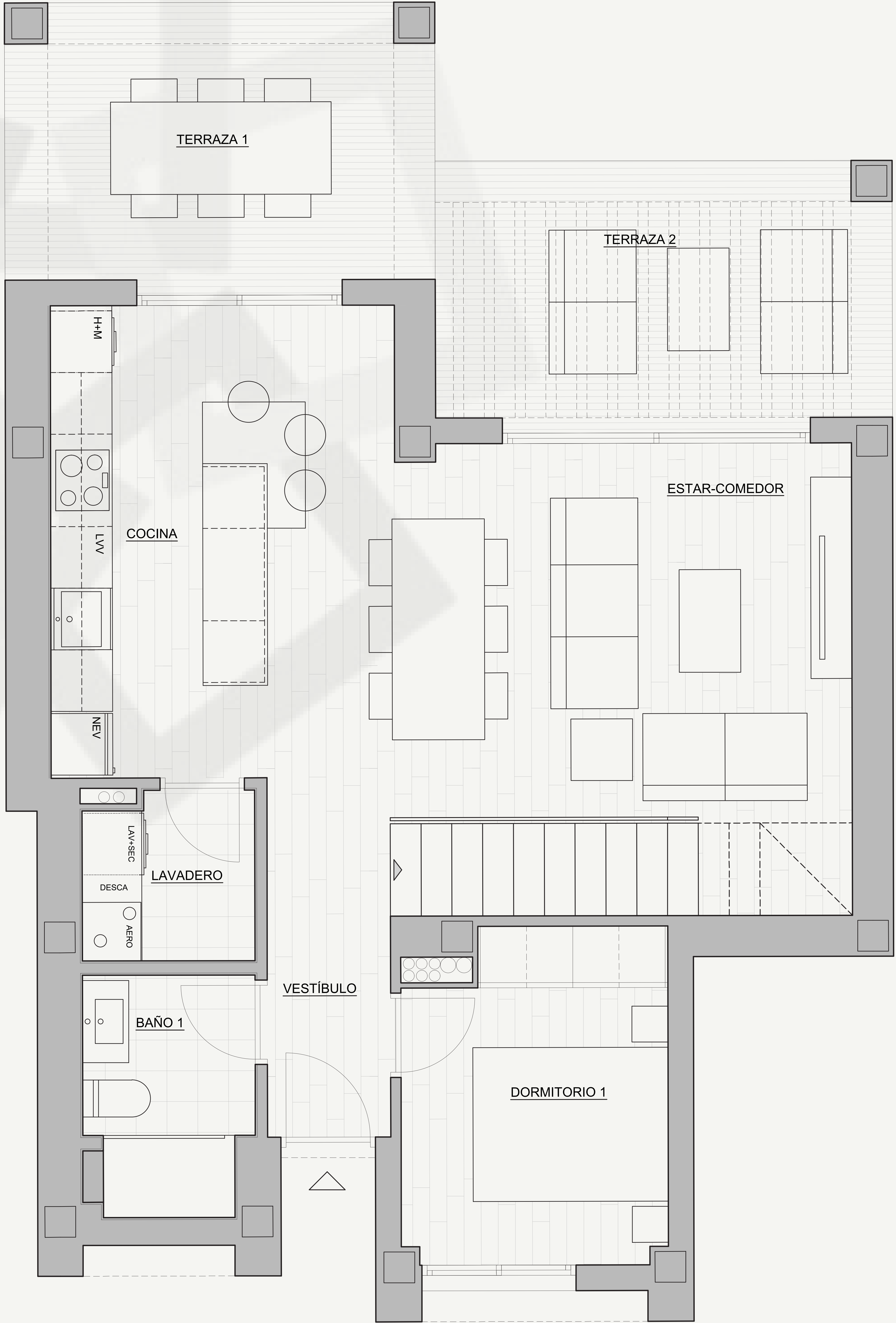
PLANTA BAJA
