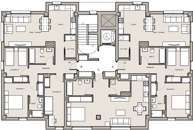
Planta TIPO (1º, 2º, 3º Y 4º)
