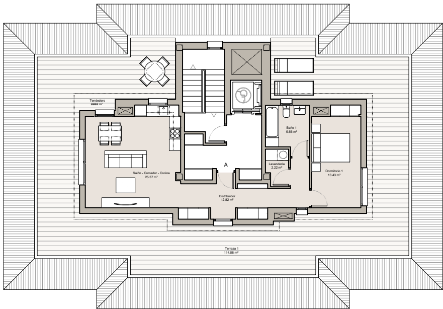
Planta Ático
