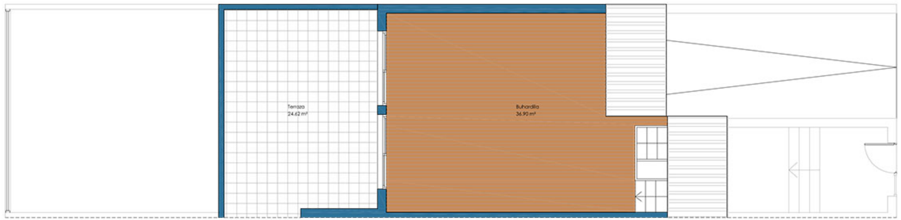
PLANTA 2º SUP. ÚTIL 36.90 m 2 SUP. CONSTRUIDA 53.44 m 2
